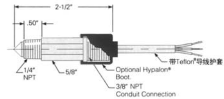
外形尺寸
